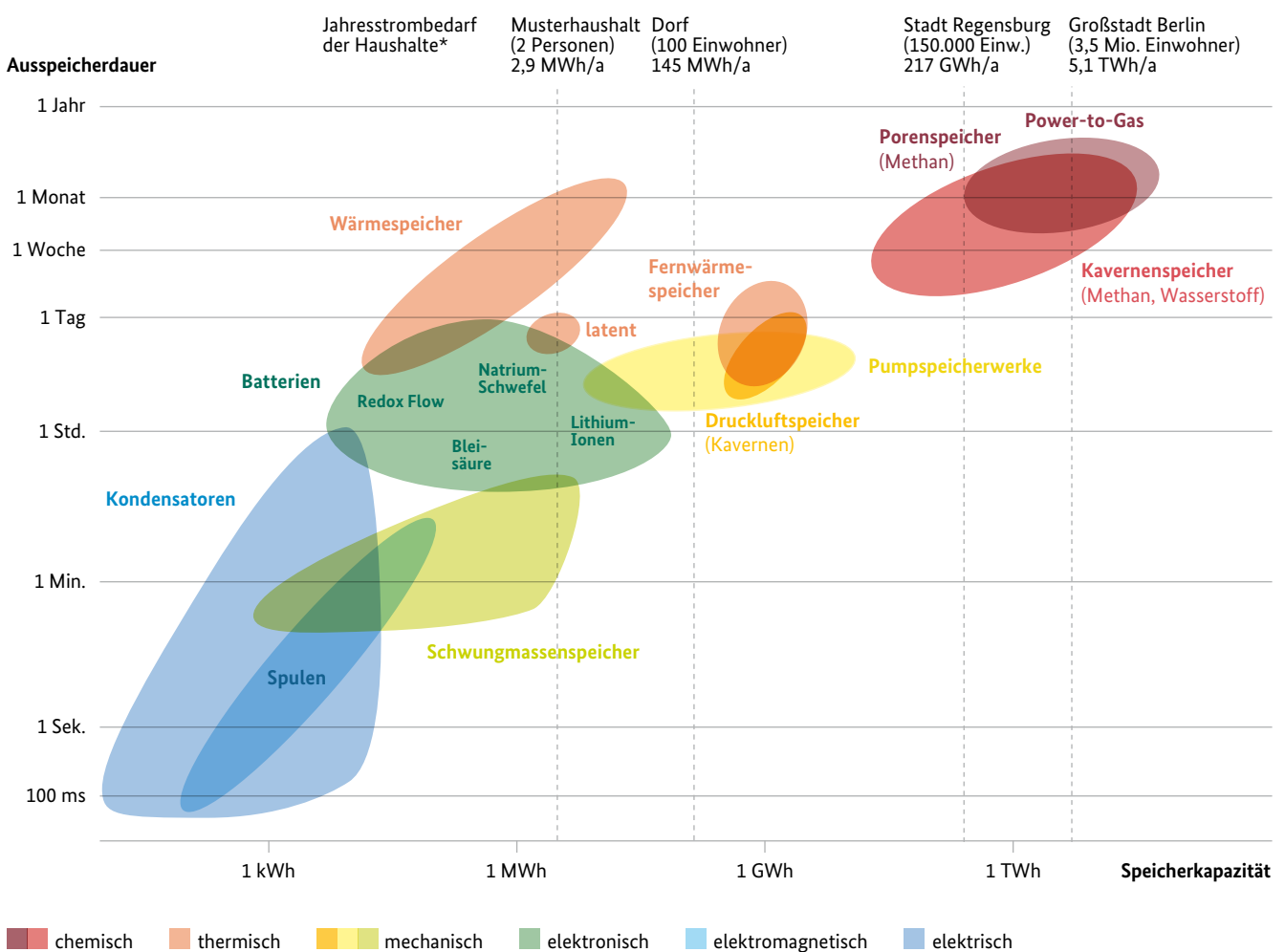
Abb. 10: Energiespeicher nach Ausspeicherdauer und Speicherkapazität
