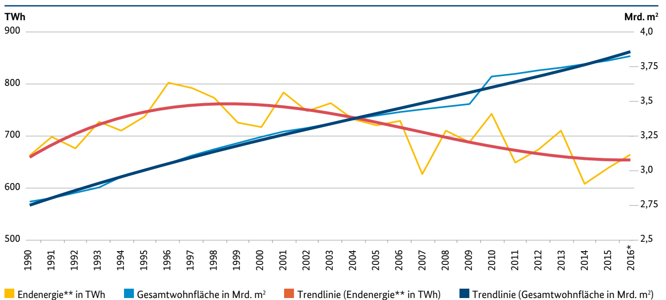
Abb. 8.2: Endenergieverbrauch der privaten Haushalte für Wohnen: Entwicklung des Endenergieverbrauchs insgesamt, sowie der Gesamtwohnfläche
